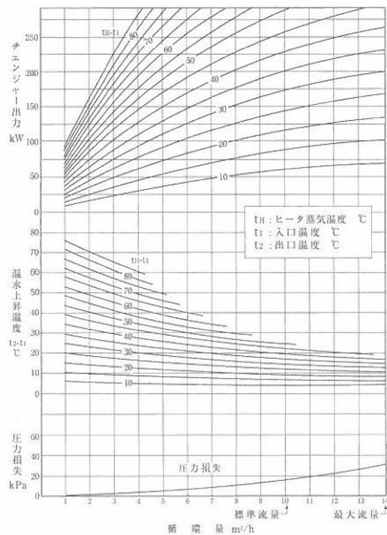
■ MFV-F400～1000 ステンレス製2回路-2パス
