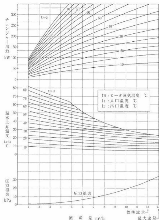
■ RKV-F300-HH 2 回路-2 パス
