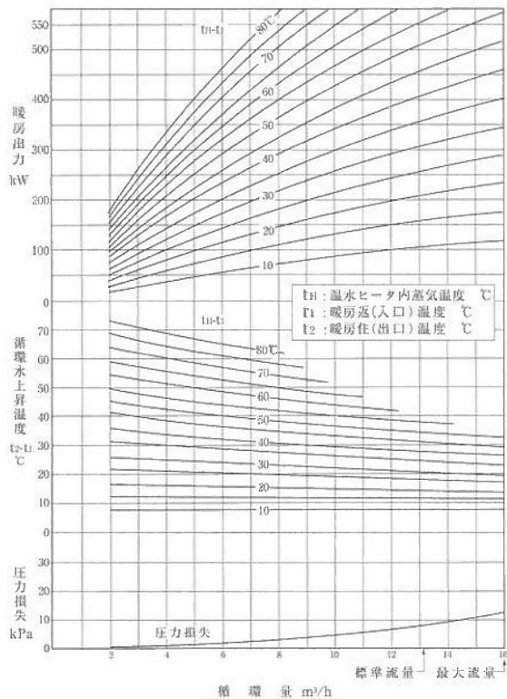
■ MFV-F400～1000 銅製2パス
