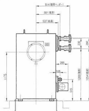
■油だきヒータ外形図
