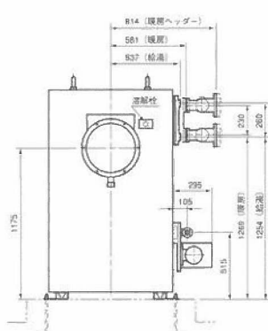
●LGXL-F-Hバーナ
