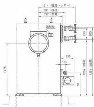
●MG-F-Hバーナ
