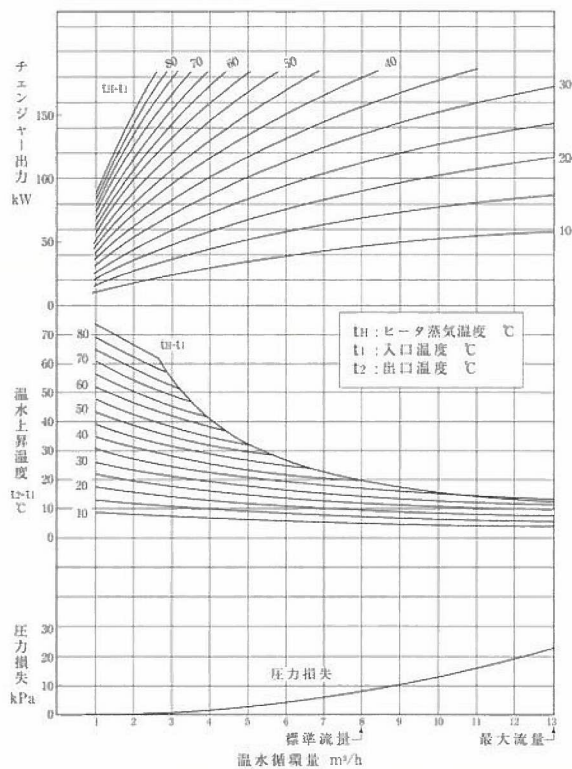
■ RKV-F160-HH 2 回路-2 パス
