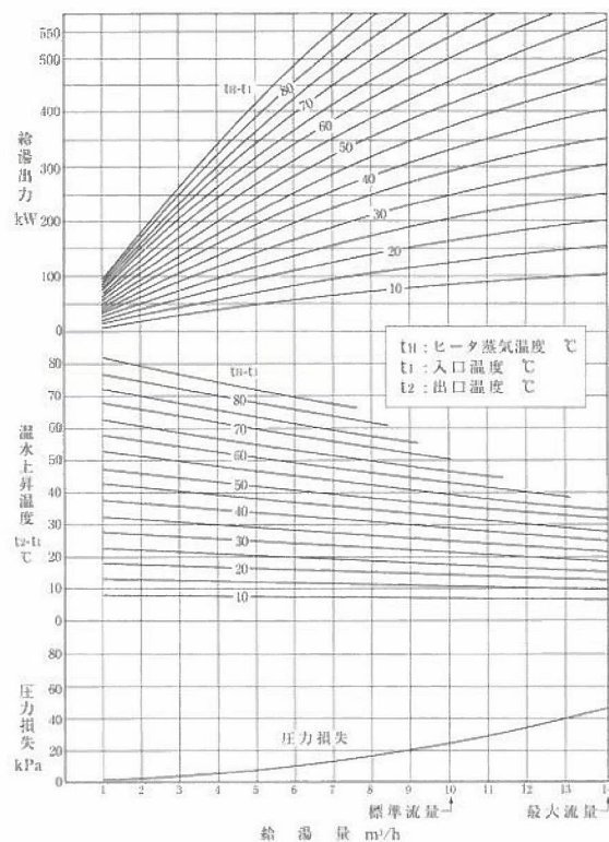
■ MFV-F400～1000 ステンレス製4パス
