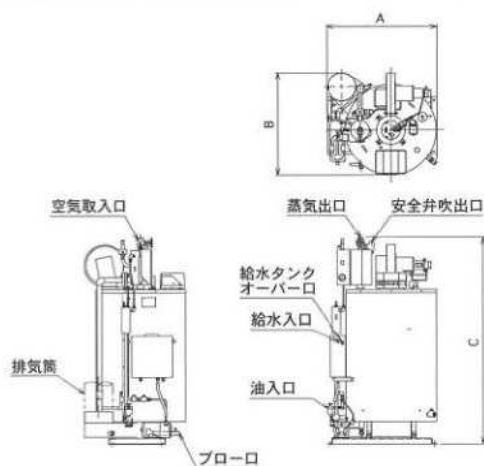
SAK 寸法図、性能・仕様表
